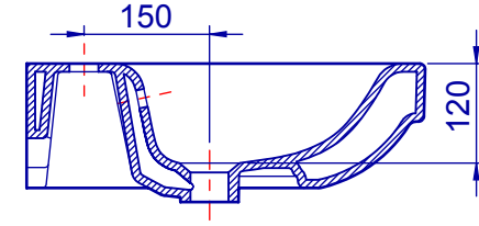
A-A KESİTİ
