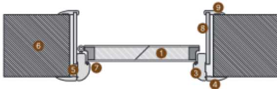
montaj ușă + perv. 12x65 + contratoc + perv.12x60
