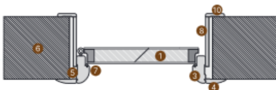
montaj ușă + perv. 12x65 + contratoc + perv.8x60
