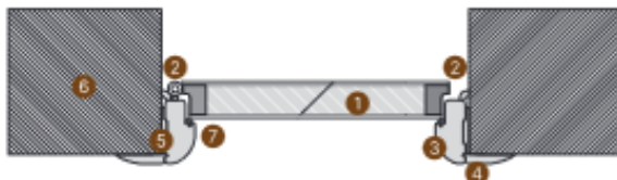
montaj ușă + perv. 12x65 + baghetă toc
